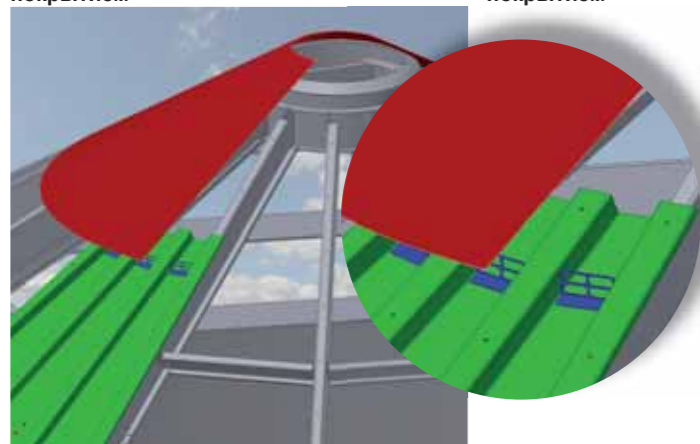
Защита от дождя и птиц. Наклон крыши 30° вместо 25°
